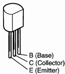
KSA916
